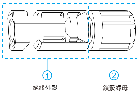
圖 5.6 正極連接器
