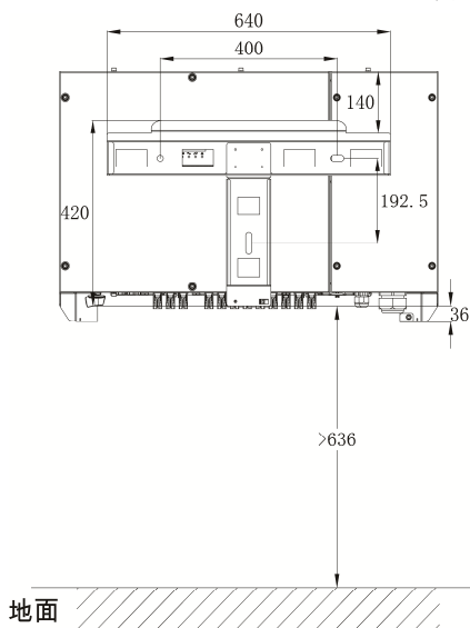
圖 4.8 附件包壁掛支架尺寸圖(單位：mm)
