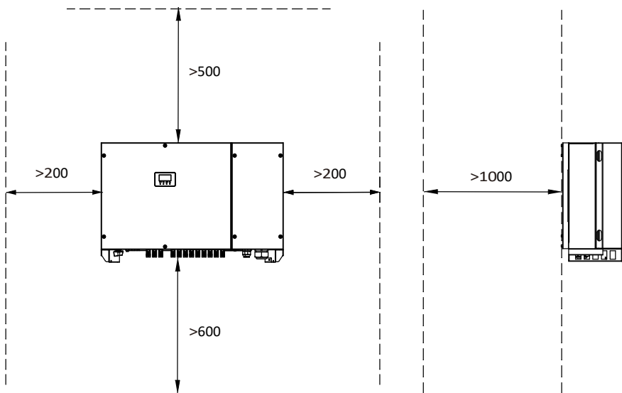
圖 4.3 安裝周圍空間要求(單位：mm)
