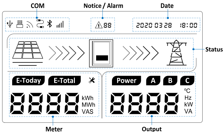
圖 8.2 LCD 螢幕
