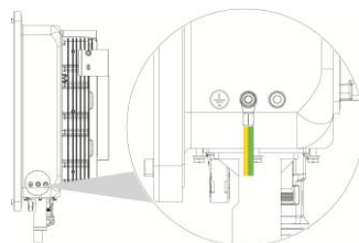
圖 5.4 變流器外部接地螺絲孔位置
