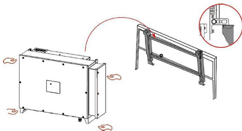
圖 4.11 變流器安裝於壁掛支架上
