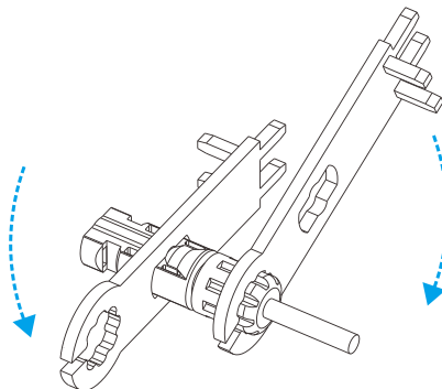
圖 5.10 鎖緊連接器
