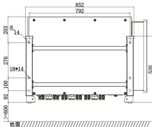
圖 4.9 附件包壁掛支架尺寸圖(單位：mm)
