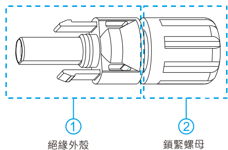
圖 5.7 負極連接器
