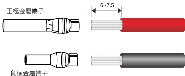
圖 5.8 直流線纜剝去絕緣層(單位：mm)
