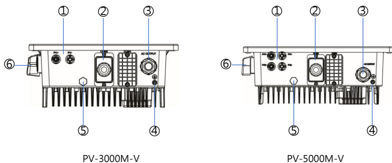
圖 2.6 PV-3000M-V/PV-5000M-V 機殼背面
