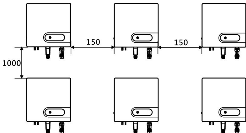
圖 4.5 上下疊安裝 (單位：mm)
