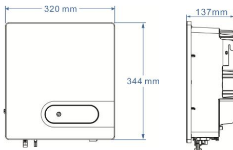
圖 2.3 PV-3000M-V 主機殼尺寸圖 (單位：mm)
