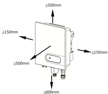
圖 4.3 安裝周圍空間要求(單位：mm)
