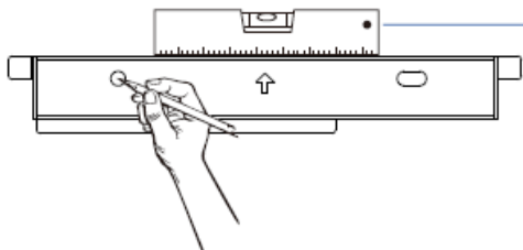
圖 4.8 壁掛支架定位
