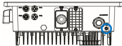
圖 5.3 變流器外部接地螺絲孔位置
