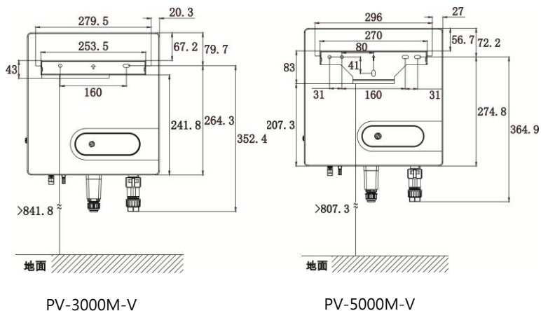
圖 4.7 壁掛支架尺寸圖(單位：mm)
