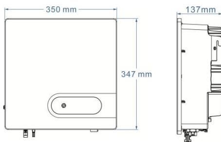
圖 2.4 PV-5000M-V 主機殼尺寸圖 (單位：mm)
