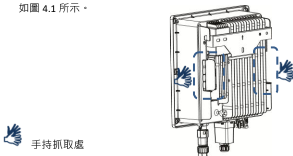
圖 4.1 變流器搬運示意圖
