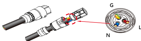
圖 5.6 輸出端連接器接線
