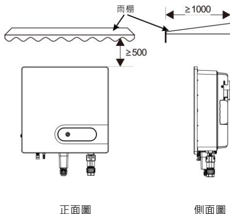
圖 4.2 有遮擋環境安裝圖(單位：mm)
