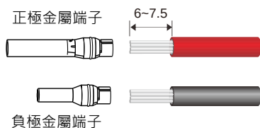
圖 5.8 直流線纜剝去絕緣層(單位：mm)
