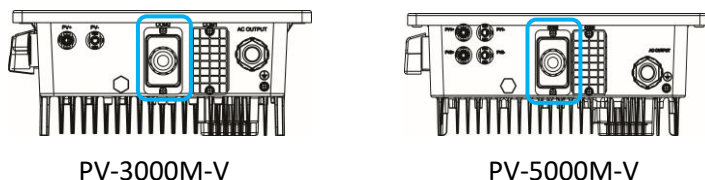
圖 5.15 RS485 接線位置
