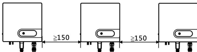
圖 4.4 一字型安裝 (單位：mm)
