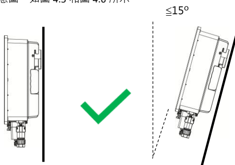
圖 4.5 正確安裝角度
