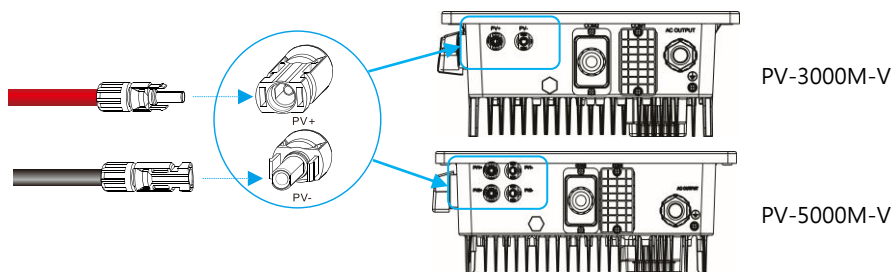
圖 5.13 接入太陽能板模組
