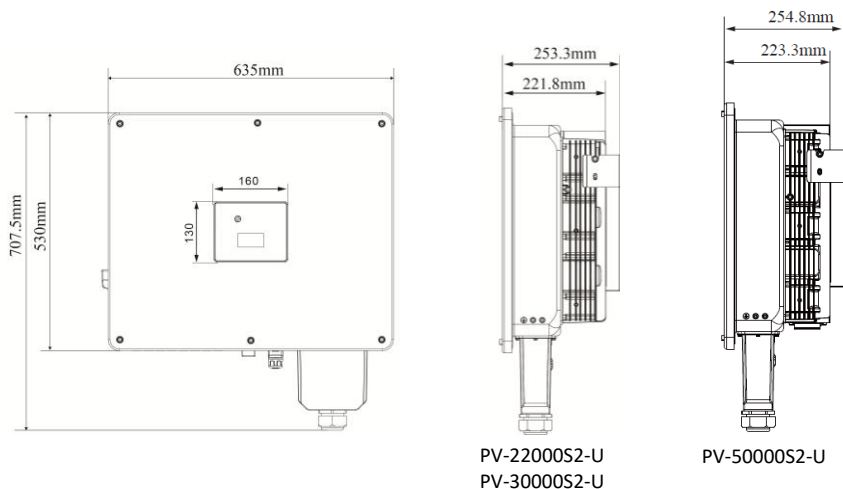
圖 2.3 主機殼尺寸圖 (單位：mm)
