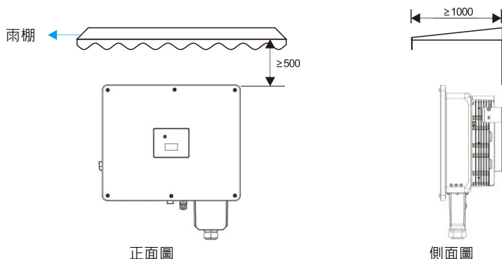
圖 4.2 有遮擋環境安裝圖(單位：mm)
