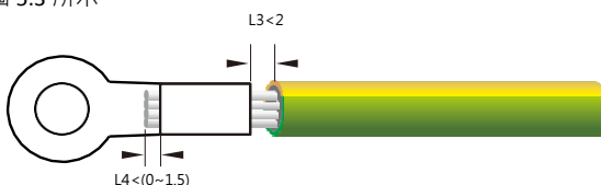
圖 5.3 壓接環型端子(單位：mm)
