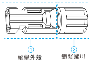
圖 5.7 正極連接器
