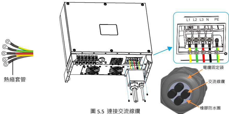
圖 5.5 連接交流線纜
