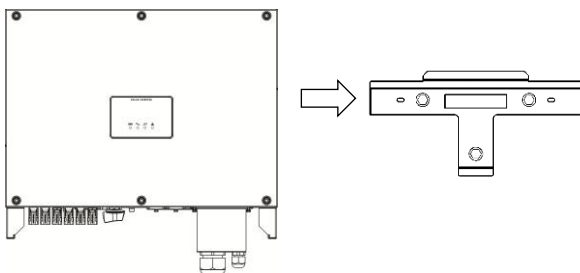
圖 4.10 將變流器掛至壁掛支架上
