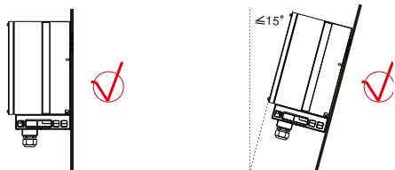
圖 4.6 正確安裝角度
