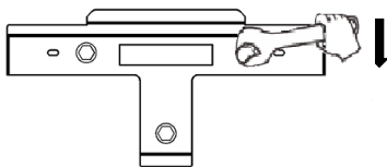
圖 4.9 壁掛支架固定
