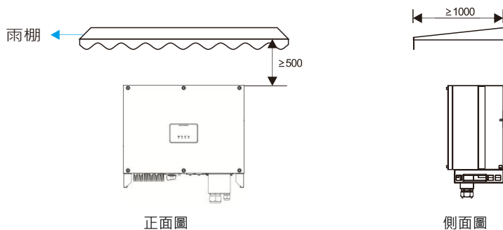
圖 4.2 有遮擋環境安裝圖(單位：mm)
