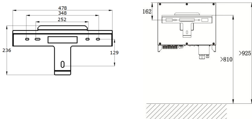
圖 4.8 附件包壁掛支架尺寸圖(單位：mm)
