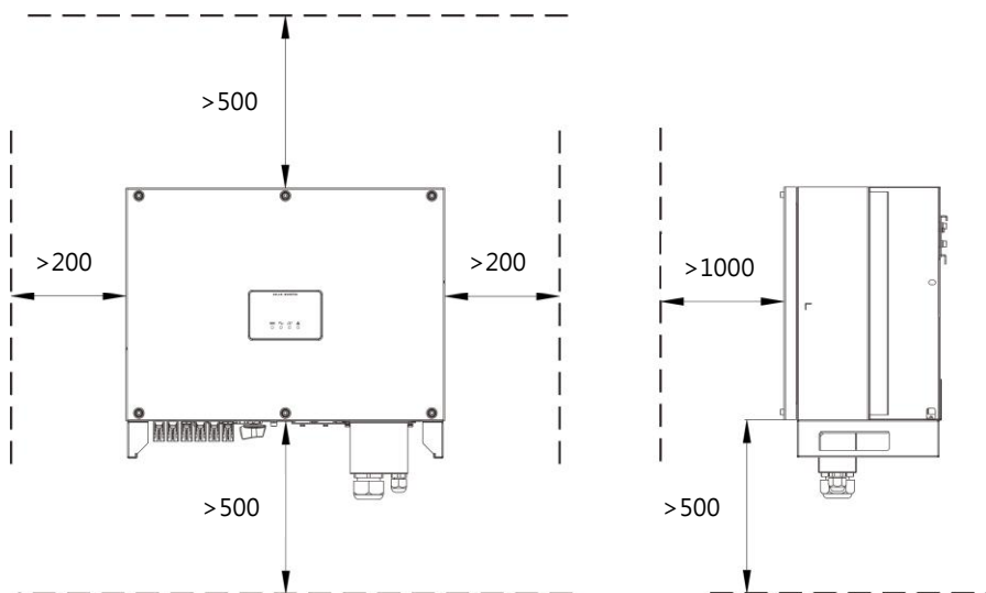
圖 4.3 安裝周圍空間要求(單位：mm)
