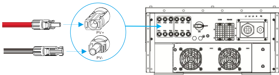
圖 5.13 接入太陽能板模組
