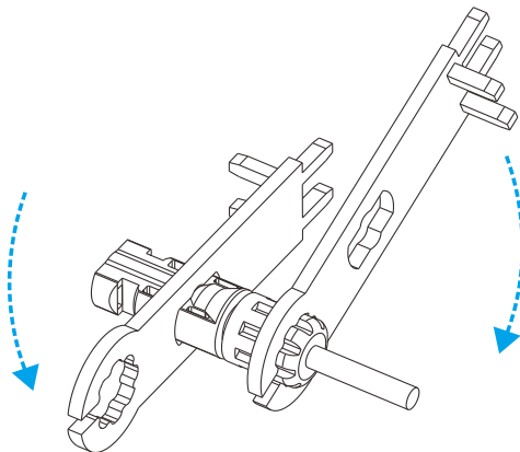
圖 5.11 鎖緊連接器
