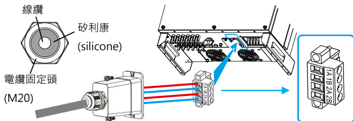
圖 5.16 RS485 端子台
