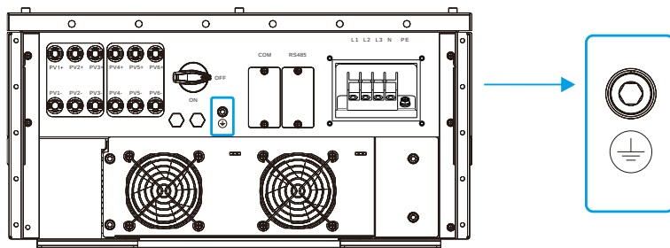
圖 5.3 變流器外部接地螺絲孔位置
