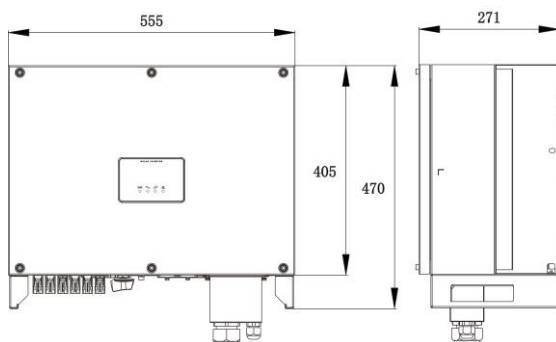
圖 2.3 主機殼尺寸圖 (單位：mm)
