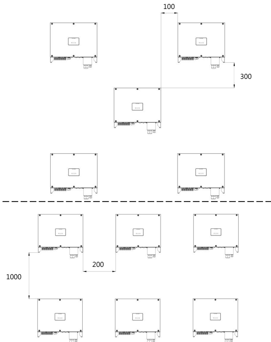
圖 4.5 品字型安裝與上下疊加型安裝(單位：mm)
