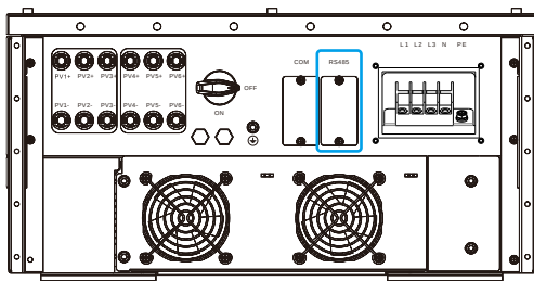
圖 5.15 RS485 接線位置
