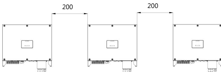
圖 4.4 一字型安裝 (單位：mm)
