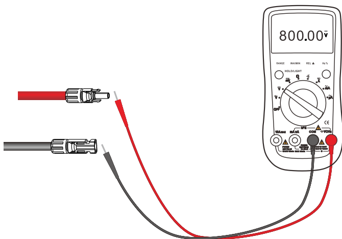
圖 5.12 檢查太陽能模組電壓
