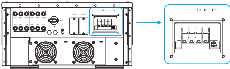
圖 5.4 交流接線位置
