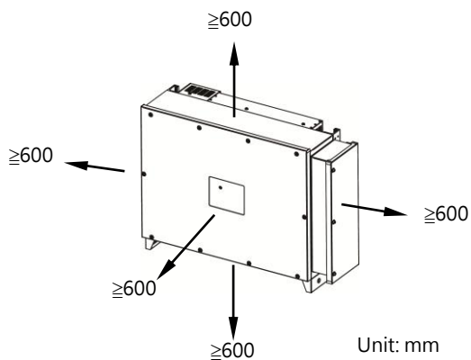
圖 4.3 安裝周圍空間要求(單位：mm)
