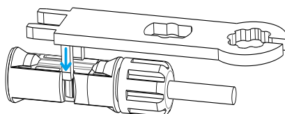
圖 9.1 拆卸直流輸入連接器
