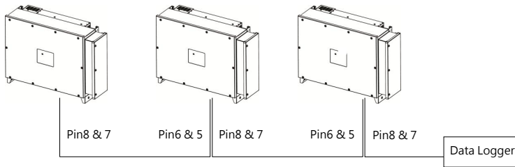
圖 5.13 標準的 RS485 連接
