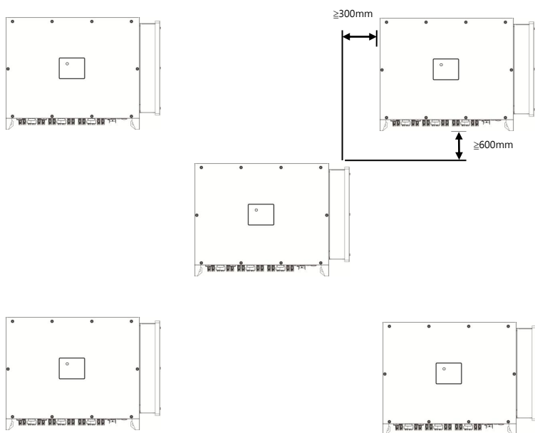
圖 4.5 品字型安裝 ( 單位：mm )
