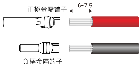
圖 5.7 直流線纜剝去絕緣層(單位：mm)
