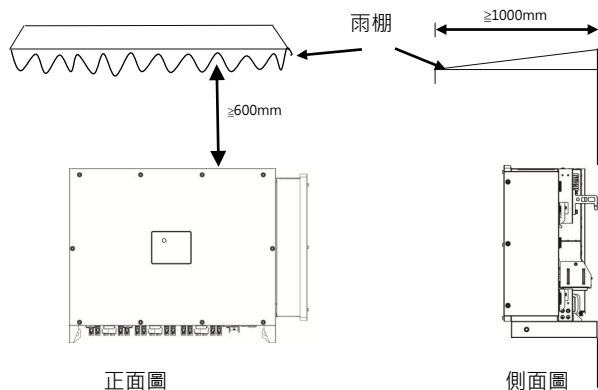
圖 4.2 有遮擋環境安裝圖(單位：mm)
