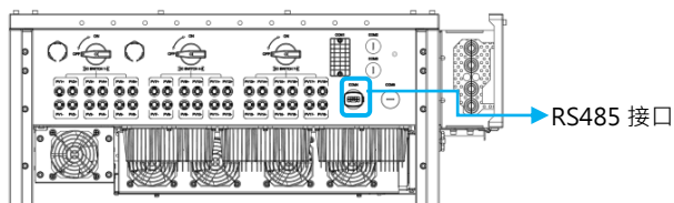
圖 5.14 RS485 接線位置
