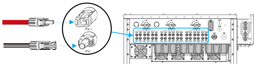
圖 5.12 接入太陽能板模組
