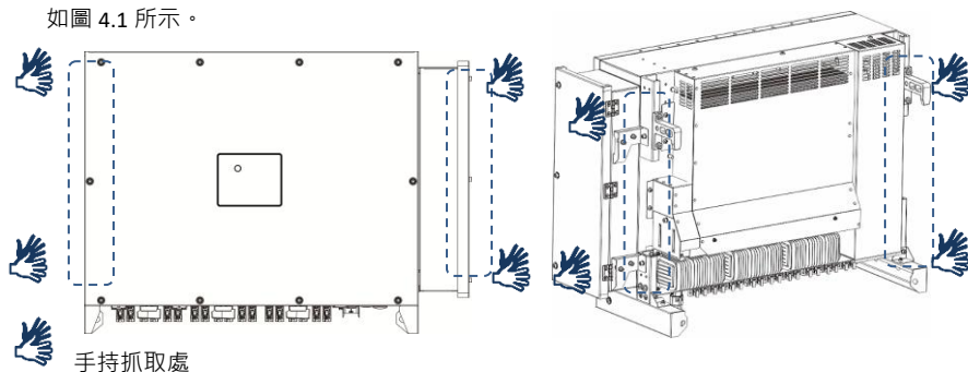
圖 4.1 變流器搬運示意圖
