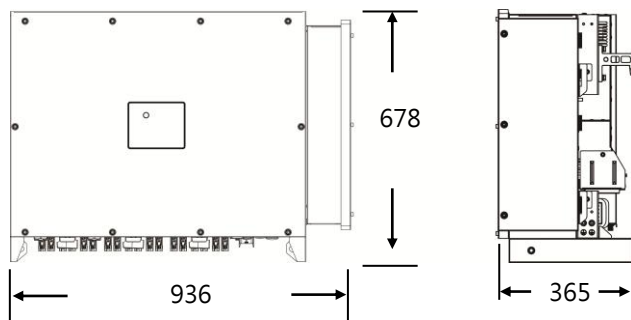
圖 2.3 PV-100KH-U/PV-110KH-U/PV-125KH-U 主機殼尺寸圖 (單位：mm)
