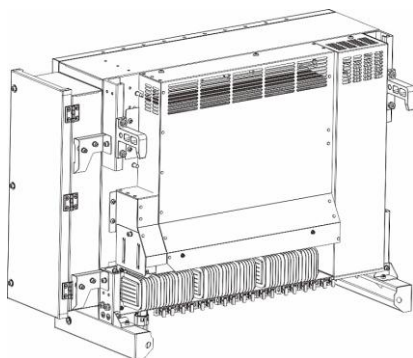
圖 2.5 PV-100KH-U/PV-110KH-U/PV-125KH-U 機殼背面
