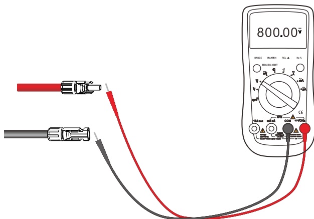
圖 5.11 檢查太陽能模組電壓
