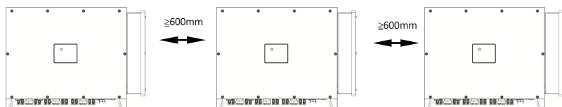
圖 4.4 一字型安裝 ( 單位：mm )
