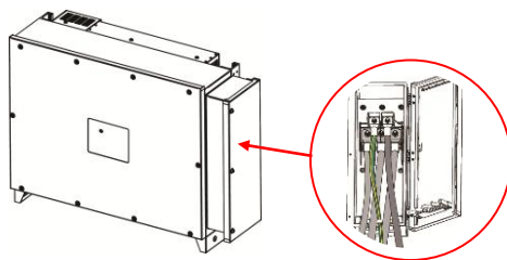
圖 5.4 交流接線位置
