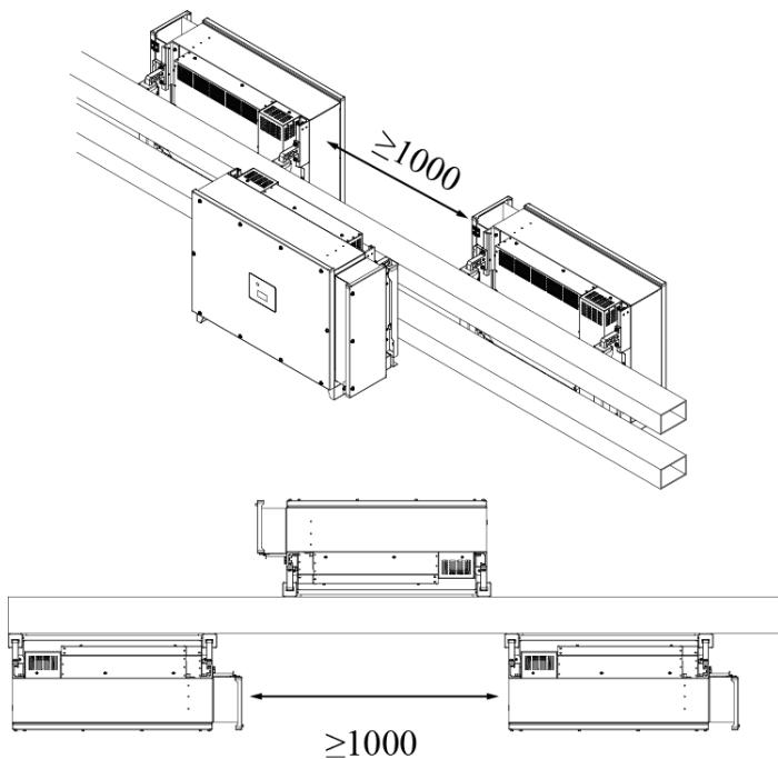
圖 4.6 背對背交錯安裝 ( 單位：mm )
