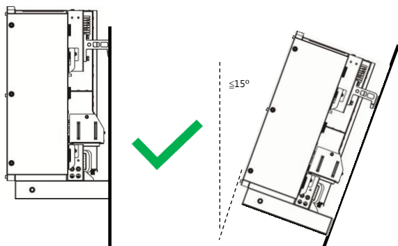
圖 4.7 正確安裝角度
