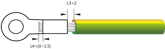
圖 5.2 壓接環型端子(單位：mm)
