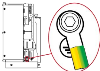
圖 5.3 變流器外部接地螺絲孔位置
