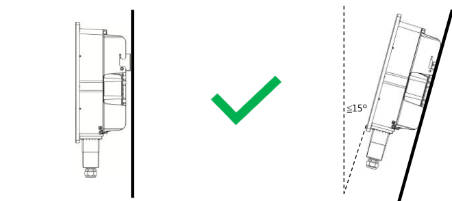
圖 4.7 正確安裝角度
