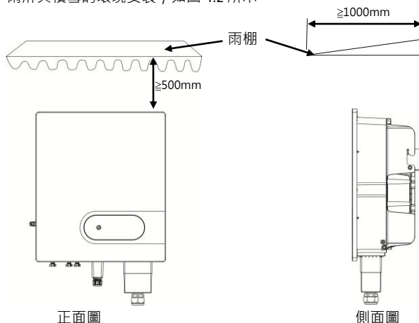
圖 4.2 有遮擋環境安裝圖(單位：mm)
