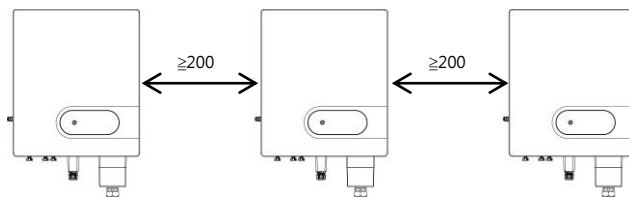
圖 4.4 一字型安裝 (單位：mm)
