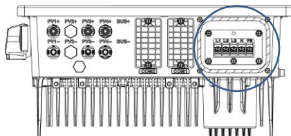
圖 5.4 交流接線位置
