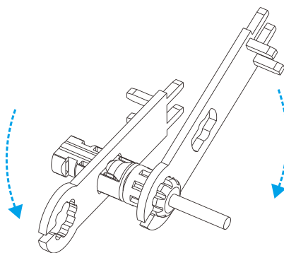
圖 5.11 鎖緊連接器
