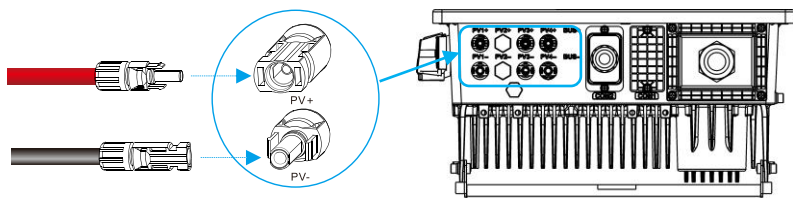
圖 5.13 接入太陽能板模組
