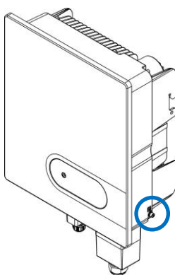
圖 5.3 變流器外部接地螺絲孔位置
