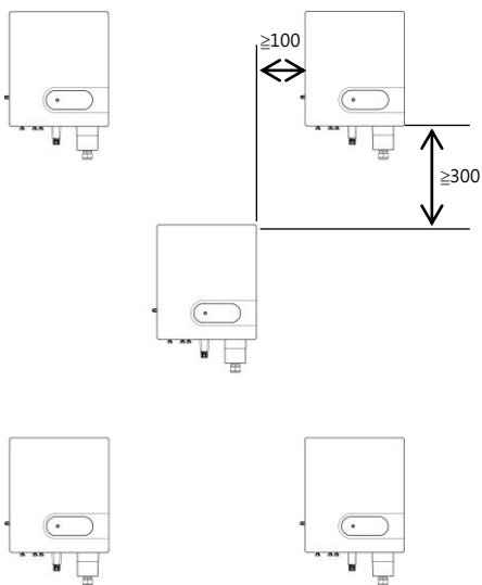
圖 4.6 品字型安裝 ( 單位：mm )
