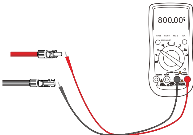
圖 5.12 檢查太陽能模組電壓
