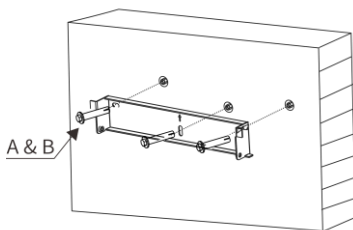
圖 4.12 壁掛支架固定
