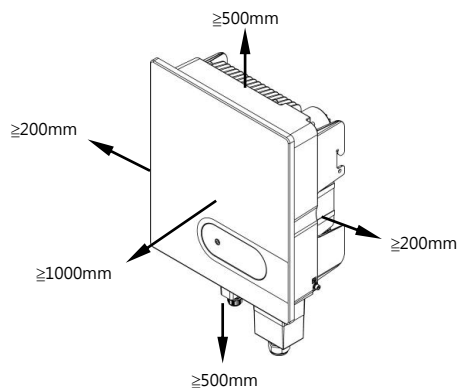
圖 4.3 安裝周圍空間要求(單位：mm)
