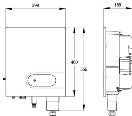
圖 2.3 PV-10000S-U/PV-15000S-U 主機殼尺寸圖（單位：mm）
