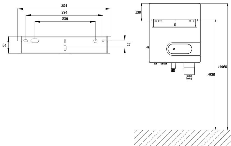
圖 4.9 附件包壁掛支架尺寸圖(單位：mm)
