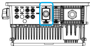
圖 5.15 RS485 接線位置
