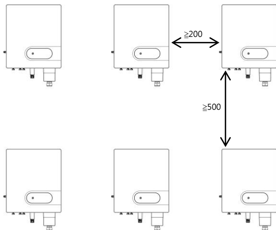
圖 4.5 上下疊安裝 ( 單位：mm )
