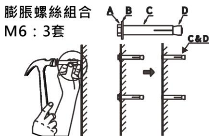
圖 4.11 膨脹螺絲使用
