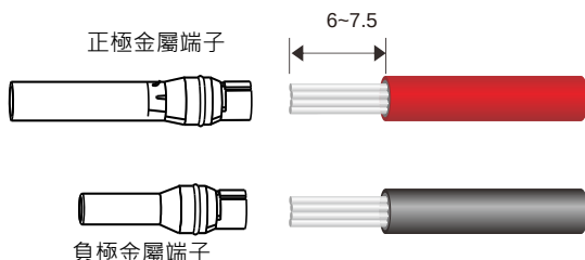
圖 5.8 直流線纜剝去絕緣層(單位：mm)
