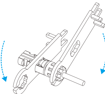
圖 5.11 鎖緊連接器
