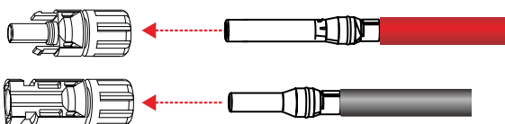
圖 5.10 插入連接器
