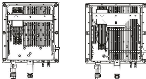
圖 2.6 PV-3000M-V/PV-5000M-V 機殼背面
