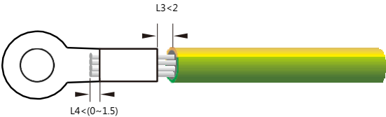
圖 5.3 壓接環型端子(單位：mm)
