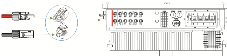
圖 5.14 接入太陽能板模組
