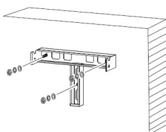
圖 4.10 壁掛支架固定
