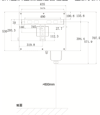
圖 4.9 附件包壁掛支架尺寸圖(單位：mm)
