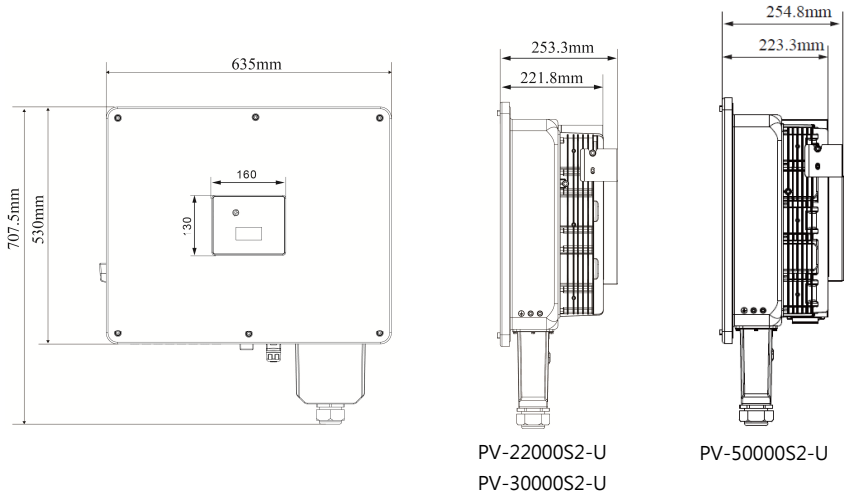
圖 2.3 主機殼尺寸圖（單位：mm）
