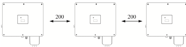
圖 4.5 一字型安裝 ( 單位 : mm )
