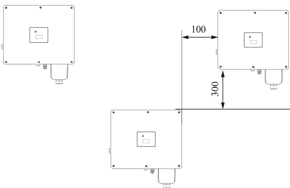
圖 4.5 一字型安裝 ( 單位 : mm )
