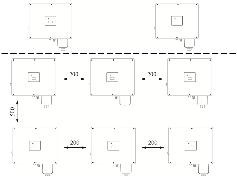
圖 4.6 品字型安裝與上下疊加型安裝(單位 : mm)
