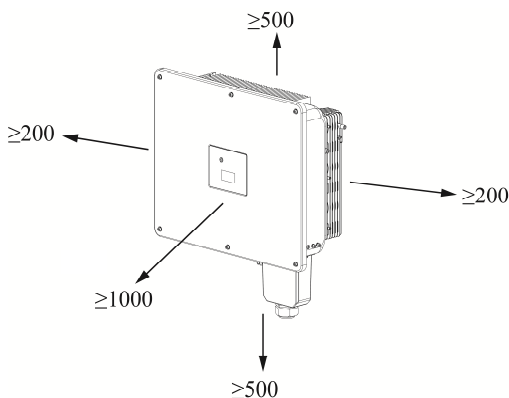
圖 4.3 PV-22000S2-U / PV-30000S2-U 安裝周圍空間要求(單位：mm)
