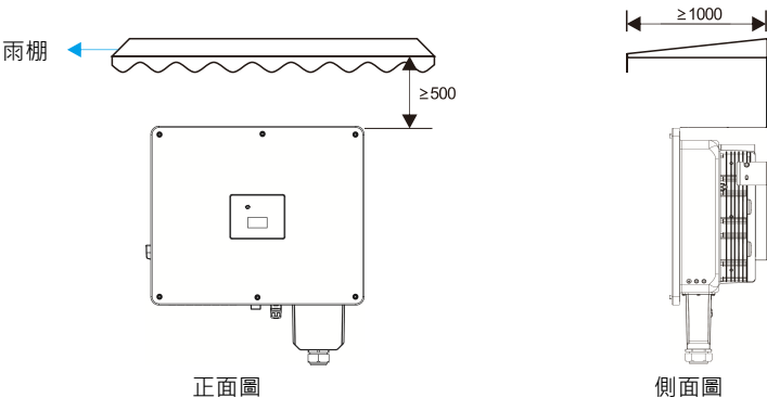
圖 4.2 有遮擋環境安裝圖(單位：mm)
