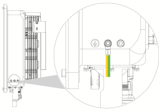
圖 5.4 變流器外部接地螺絲孔位置
