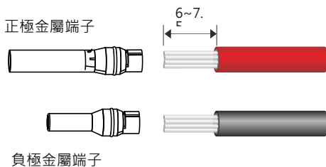
圖 5.9 直流線纜剝去絕緣層(單位：mm)
