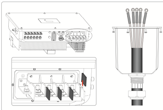
圖 5.6 連接交流線纜
