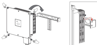
圖 4.11 將變流器掛至壁掛支架上
