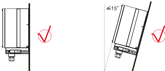
圖 4.7 正確安裝角度
