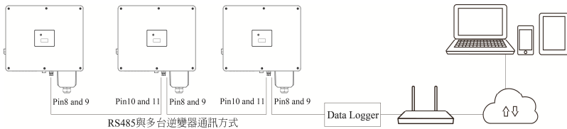
圖 5.15 標準的 RS485 連接
