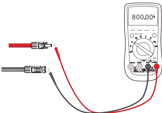
圖 5.13 檢查太陽能模組電壓
