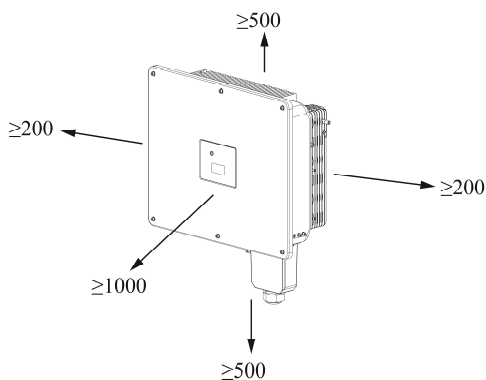
圖 4.4 PV-50000S2-U 安裝周圍空間要求(單位：mm)
