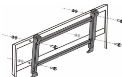
圖 4.10 壁掛支架定位
