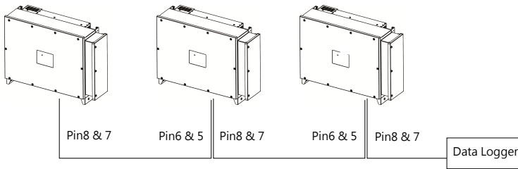
圖 5.13 標準的 RS485 連接
