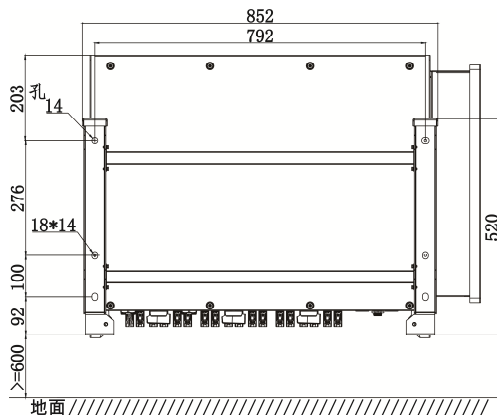
圖 4.9 附件包壁掛支架尺寸圖(單位：mm)
