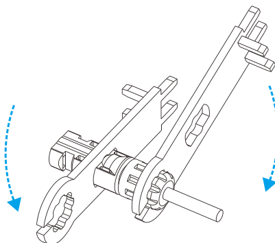
圖 5.10 鎖緊連接器
