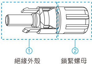
圖 5.6 負極連接器
