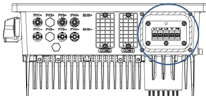
圖 5.4 交流接線位置
