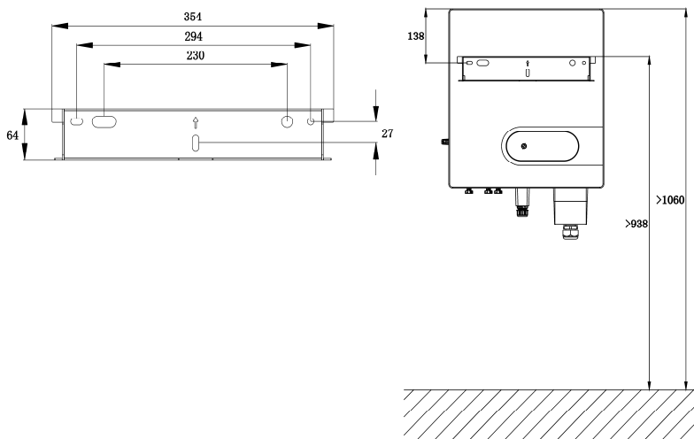
圖 4.9 附件包壁掛支架尺寸圖(單位：mm)
