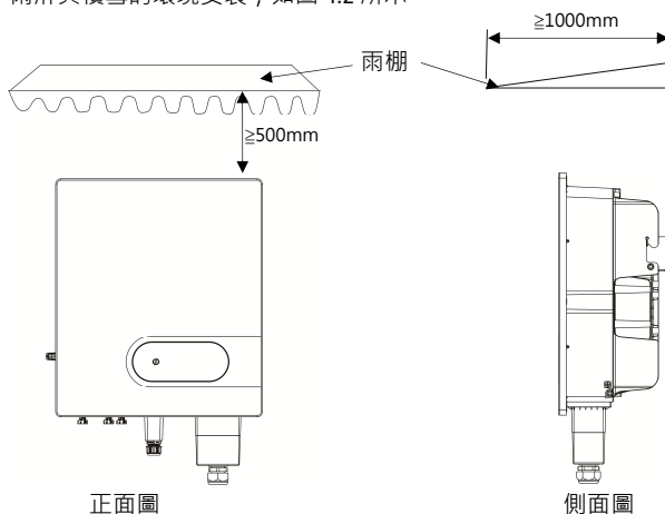
圖 4.2 有遮擋環境安裝圖(單位：mm)
