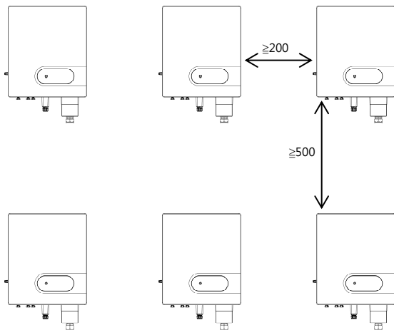
圖 4.5 上下疊安裝 ( 單位：mm )
