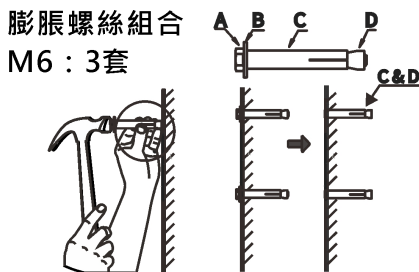
圖 4.11 膨脹螺絲使用
