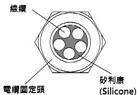
圖 5.5 連接交流線纜
