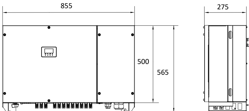
圖 2.3 PV-6000T-U/PV-7500T-U/PV-6000H-U/PV-7500H-U 主機殼尺寸圖 (單位：mm)
