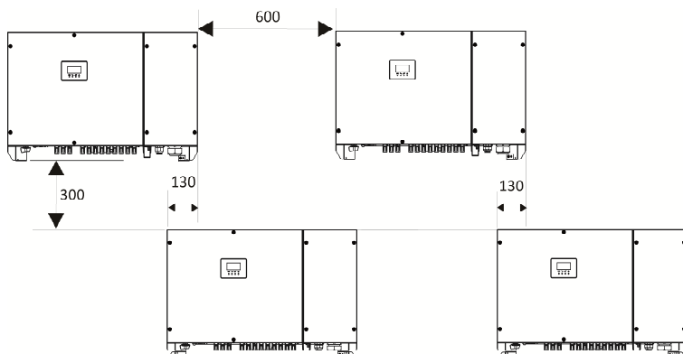
圖 4.5 上下疊加型安裝(單位：mm)
