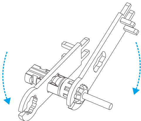
圖 5.11 鎖緊連接器
