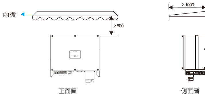
圖 4.2 有遮擋環境安裝圖(單位：mm)
