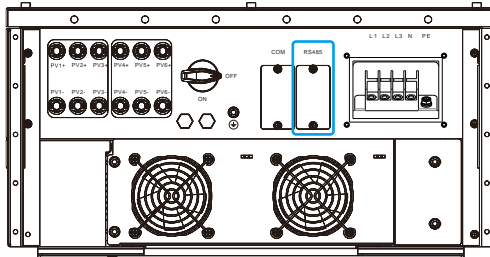
圖 5.15 RS485 接線位置
