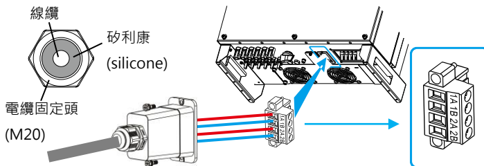
圖 5.16 RS485 端子台
