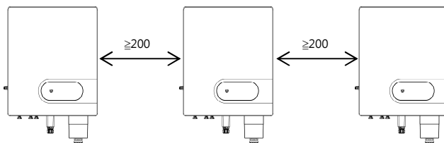
圖 4.4 一字型安裝 (單位：mm)
