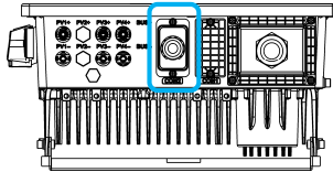
圖 5.15 RS485 接線位置
