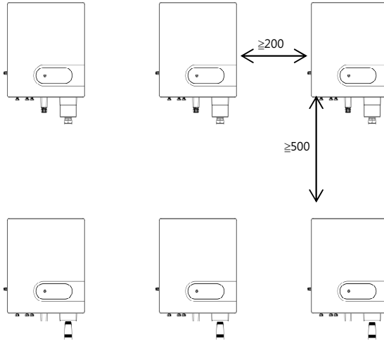
圖 4.5 上下疊安裝 (單位：mm)
