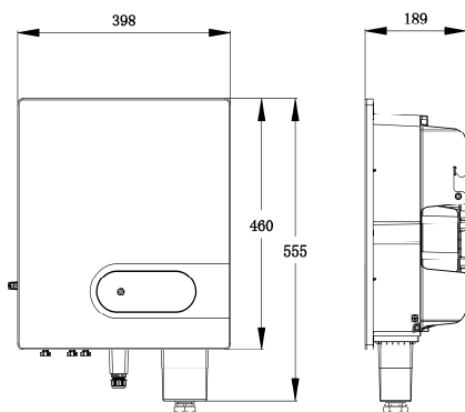
圖 2.3 PV-10000S-U/PV-15000S-U 主機殼尺寸圖 (單位：mm)
