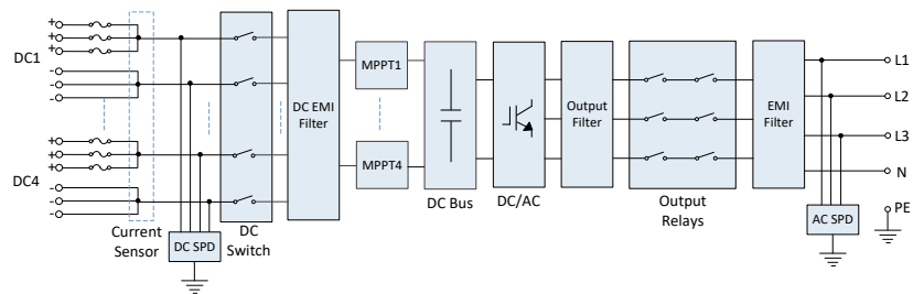
電氣方塊圖
