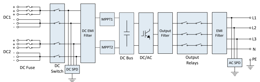
PV-30000S-U 電氣方塊圖
