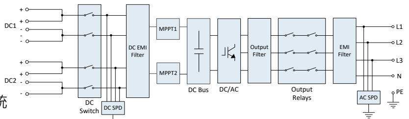
PV-30000S-U 電氣方塊圖
