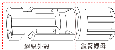
圖 5.8 正極連接器
