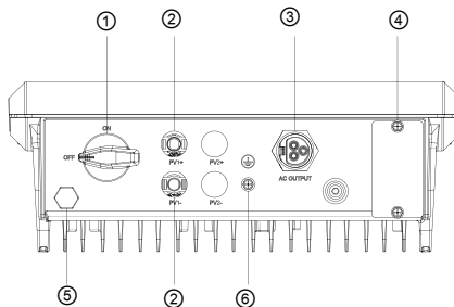
圖 2.8 PV-5000S-HV 主機介面
