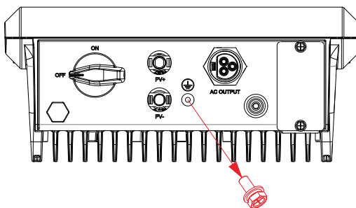
圖 5.3 鬆開地線螺絲
