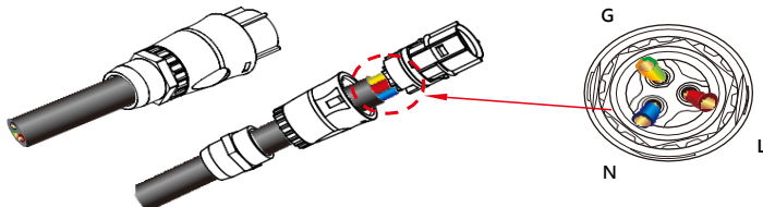
圖 5.6 輸出端連接器接線
