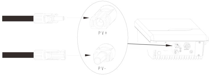
圖 5.15 接入太陽能板模組
