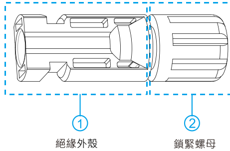
圖 5.6 正極連接器
