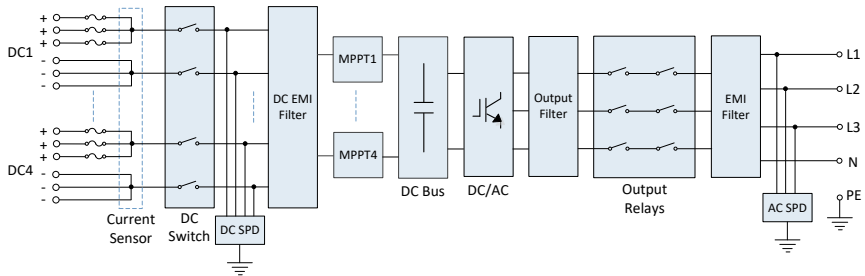
【電氣方塊圖】
