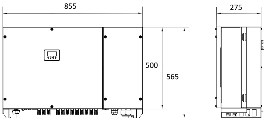
圖 2.3 PV-60000T-U/PV-75000T-U 主機殼尺寸圖 (單位：mm)
