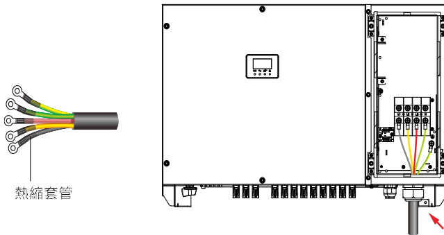
圖 5.5 連接交流線纜
