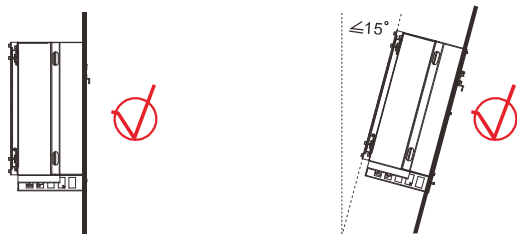
圖 4.6 正確安裝角度
