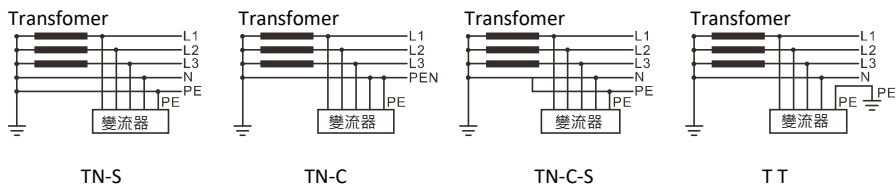
圖 2.2 本系列變流器電網系統
