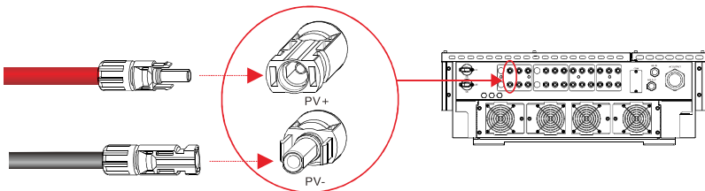
圖 5.13 接入太陽能板模組
