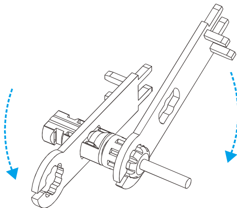
圖 5.11 鎖緊連接器
