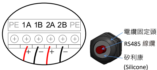
圖 5.16 RS485 端子台
