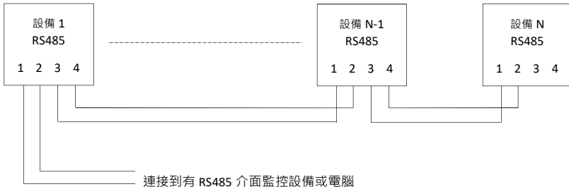
圖 5.14 標準的 RS485 連接
