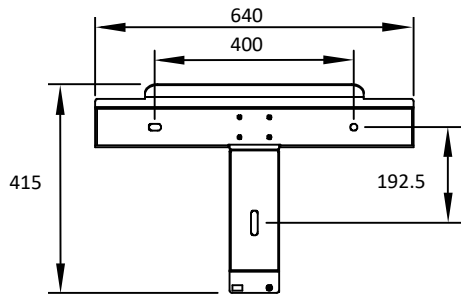
圖 4.8 附件包壁掛支架尺寸圖(單位：mm)
