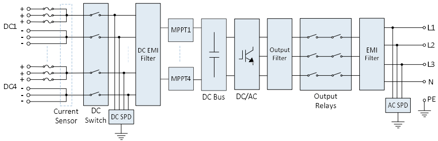
【電氣方塊圖】
