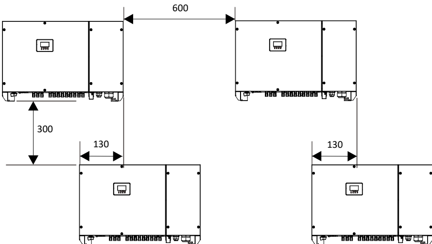
圖 4.5 上下疊加型安裝(單位：mm)
