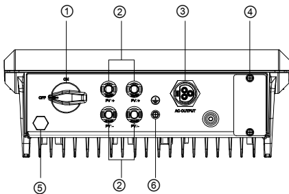
圖 2.7 PV-5000S-V 主機介面
