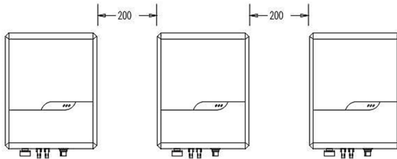
圖 4.5 一字型安裝 (單位：mm)
