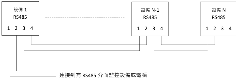
圖 5.16 標準的 RS485 連接
