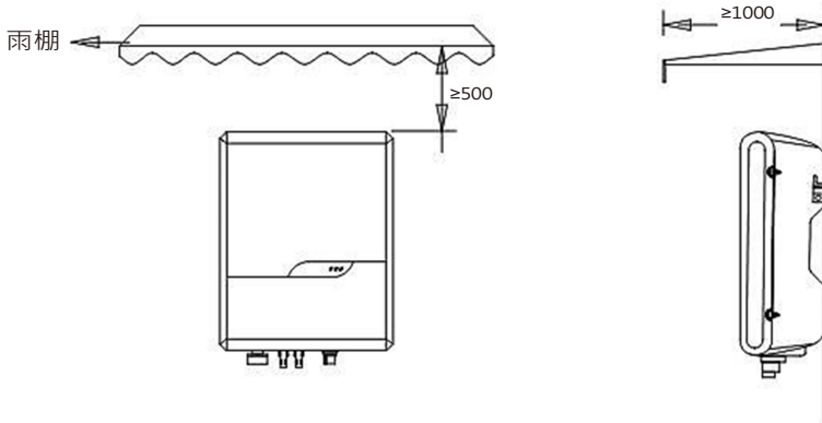
圖 4.3 有遮擋環境安裝圖 (單位：mm)
