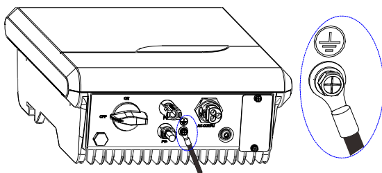
圖 5.4 鎖緊地線
