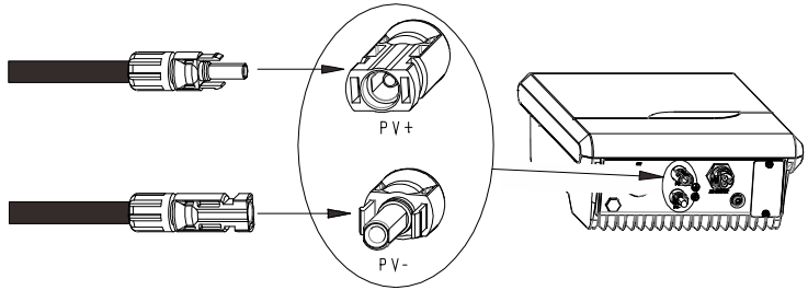
圖 5.15 接入太陽能板模組
