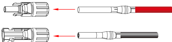
圖 5.12 插入連接器
