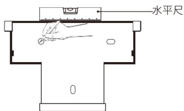
圖 4.11 標記孔位
