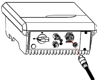
圖 5.7 交流連接器接入變流器
