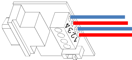
圖 5.19 連接通訊線纜
