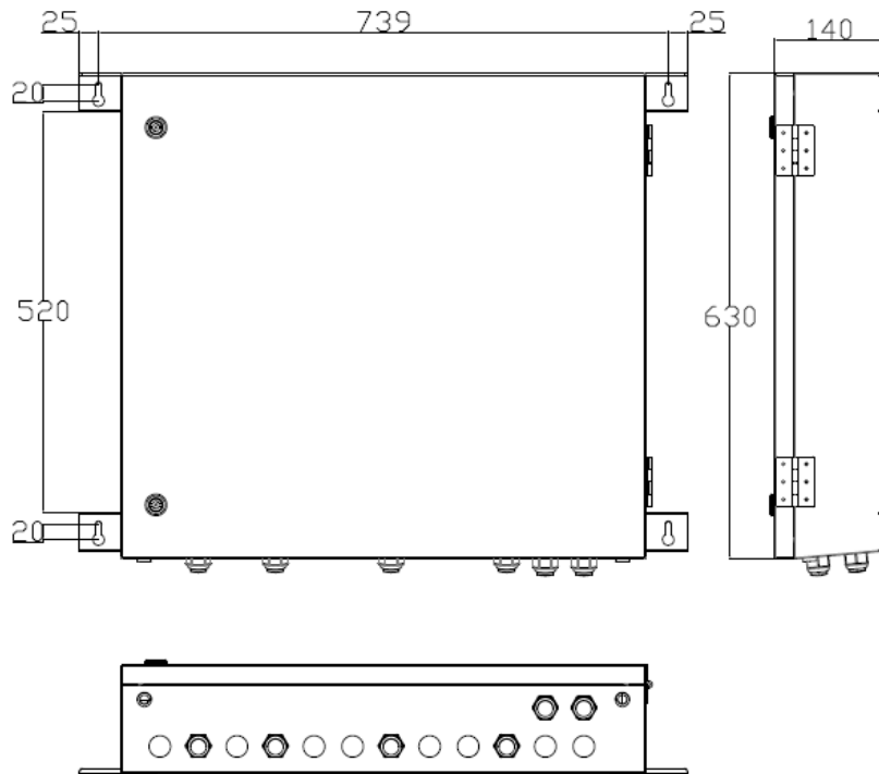
圖一：PV-1-DC-1C 尺寸
