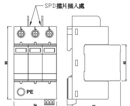
圖四：SPD擋片安裝完成示意圖
